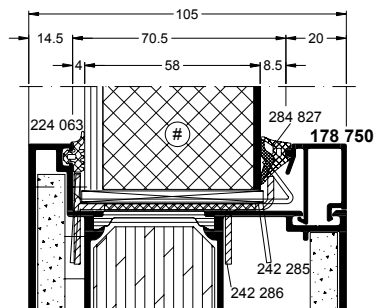
Brandschutz-Glas / Alu-Paneel
